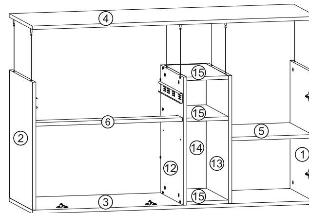
ПРАВОВОСТОРОННЯЯ СБОКА RIGHT-HANDED ASSEMBLY
